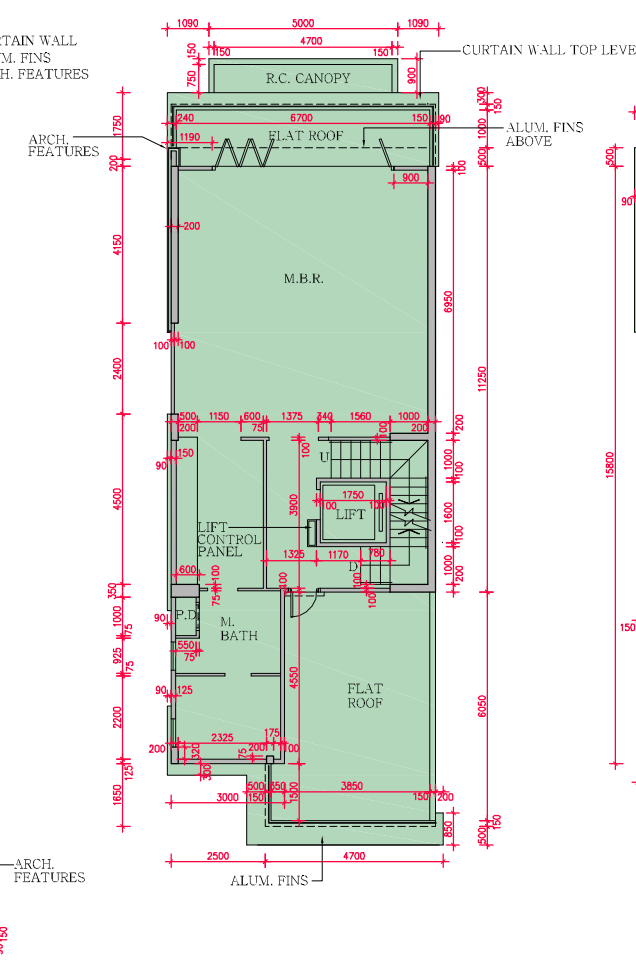
2/F PLAN 2樓平面圖
