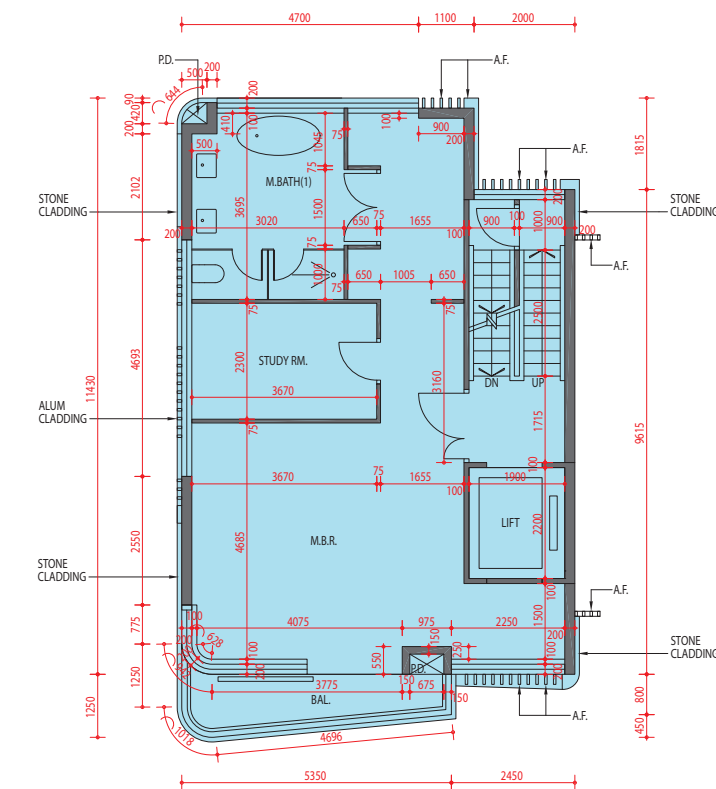
2/F Floor Plan 2樓平面圖
