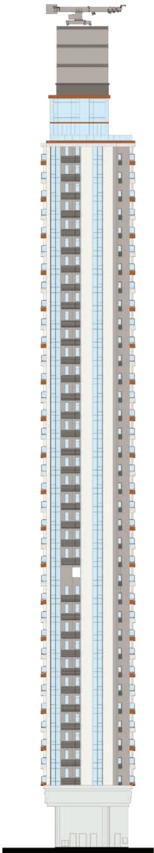
Elevation Plan 2 - Tower 1 (Tower 1B) 立面圖2 - 第1座(第1B座)
