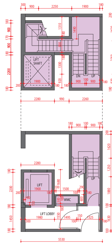
G/F Floor Plan 地下平面圖
