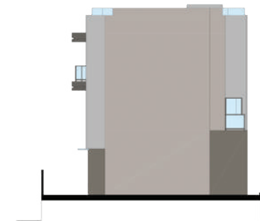
Elevation Plan D 立面圖 D
