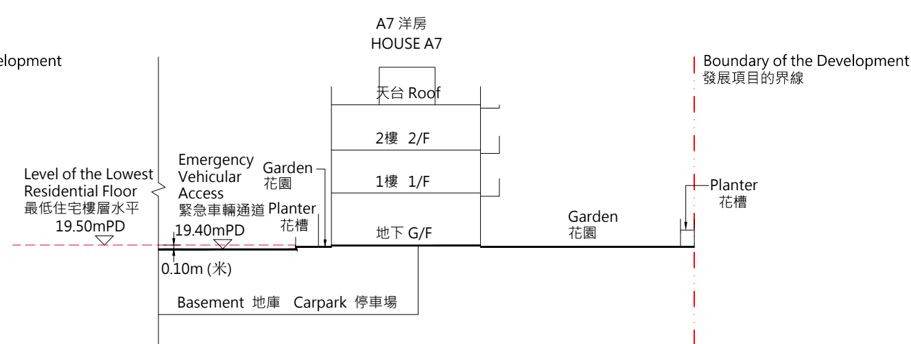
Cross-section Plan A7 橫截面圖 A7
