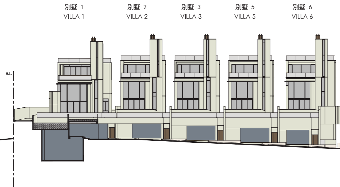
立面 E Elevation E
