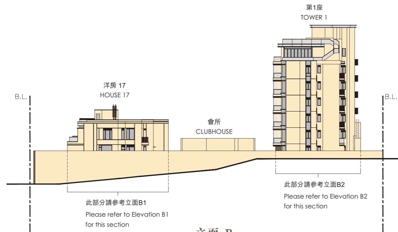
第1座 TOWER 1 立面 B Elevation B
