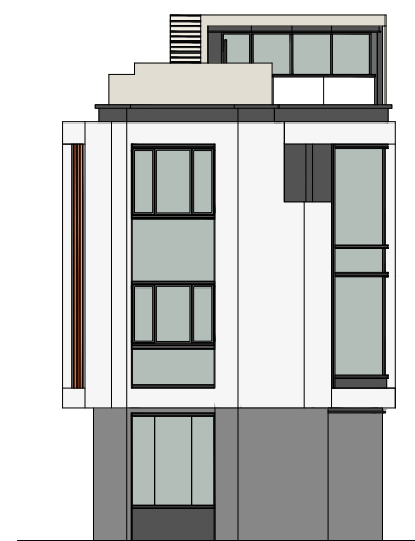
立面圖 B1 ( 適用於 A12 洋房 ) Elevation Plan B1 ( For House A12 )
