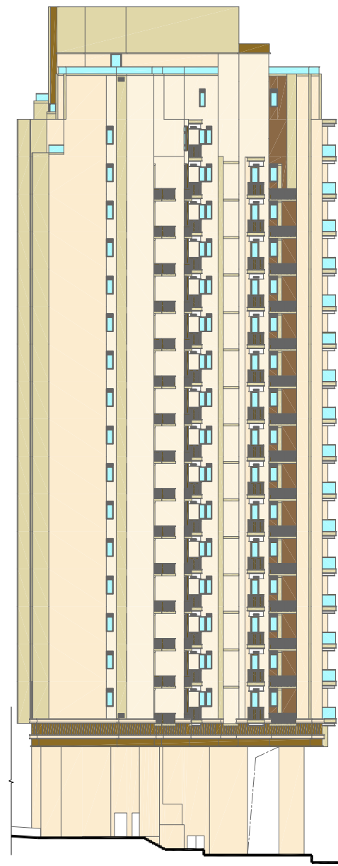
ELEVATION A 立面圖 A
