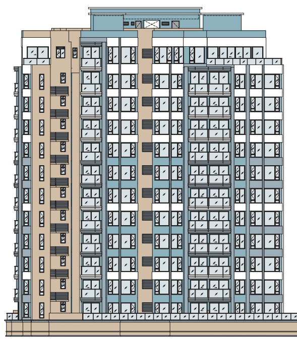
Elevation 2 立面 2
