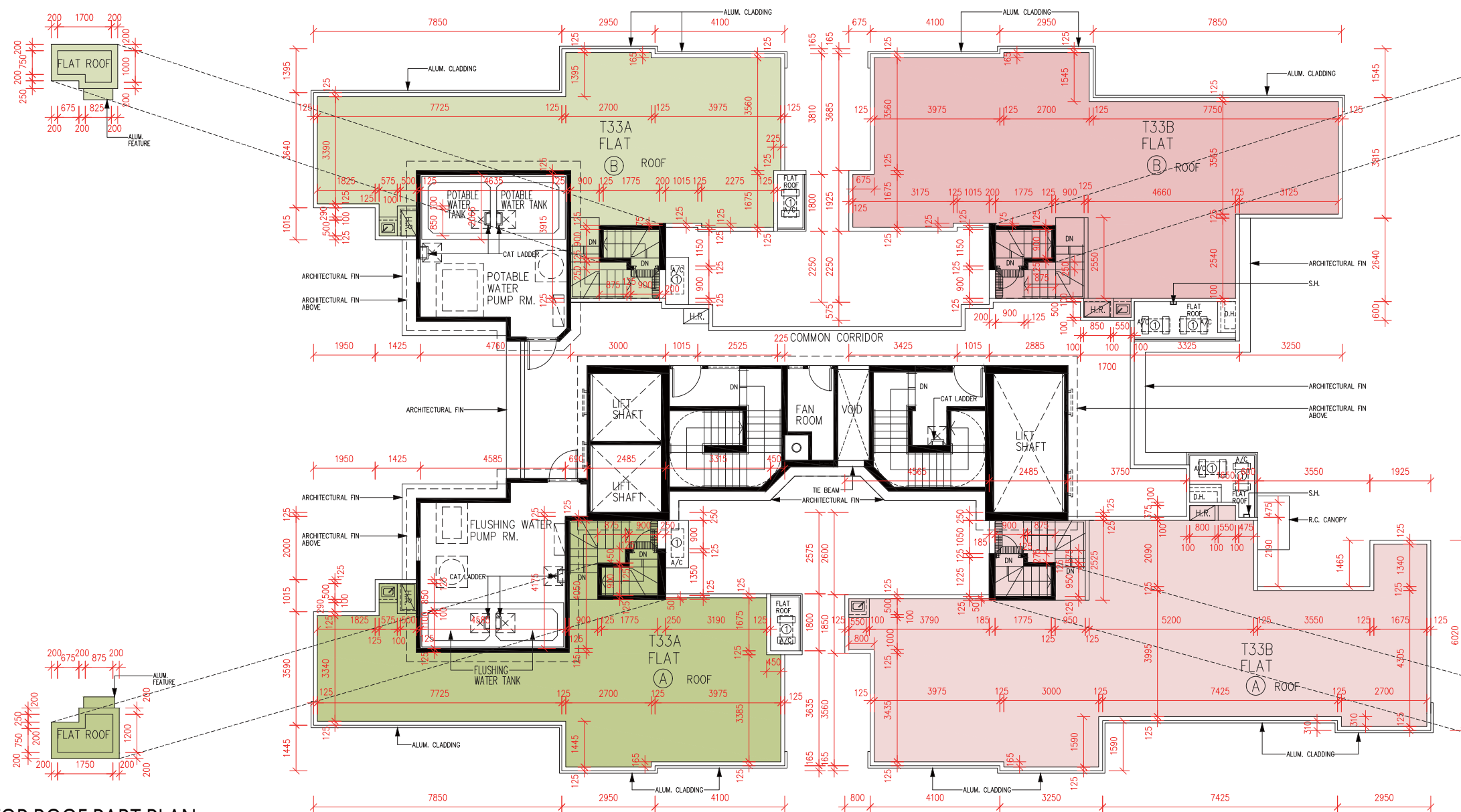
TOP ROOF PART PLAN 天台頂層局部平面圖
