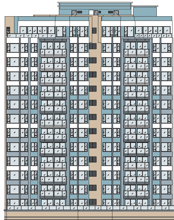
Elevation 2 立面 2
