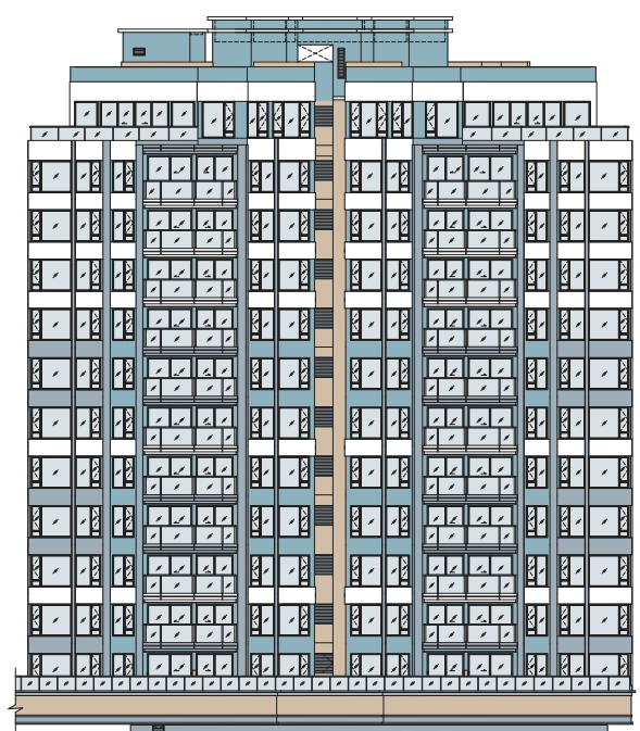
Elevation 4 立面 4
