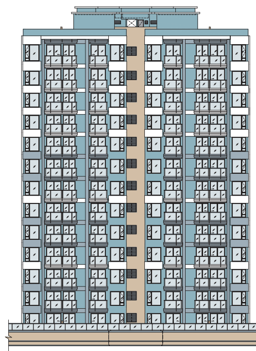
Elevation 2 立面 2
