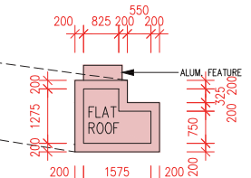
TOP ROOF PART PLAN 天台頂層局部平面圖
