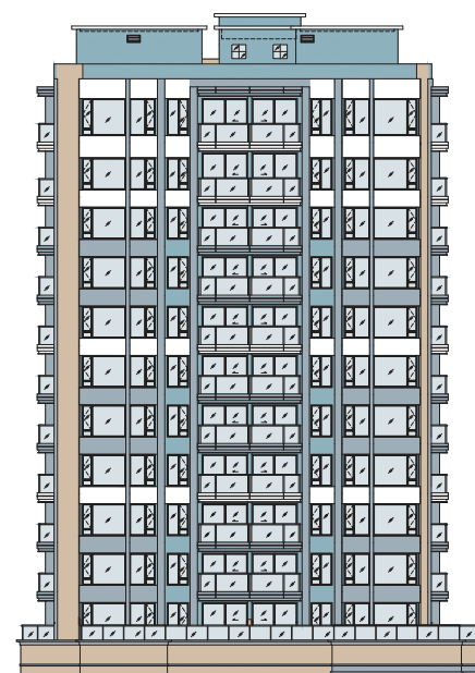
Elevation 1 立面 1
